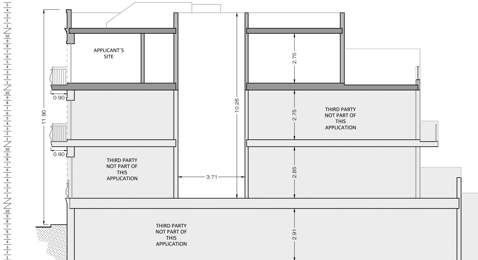
LONGITUDINAL SECTION X : X
